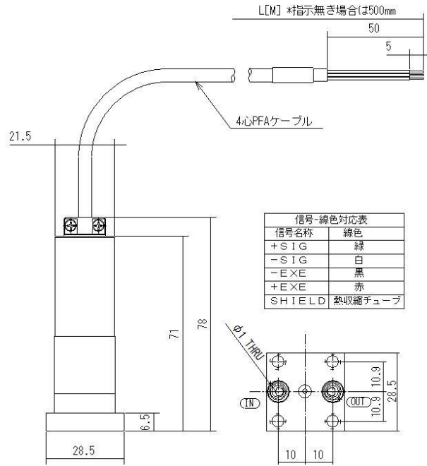
PC-302SIF-**A-HT-AN-[L]M (1.125”、Wシール仕様)
